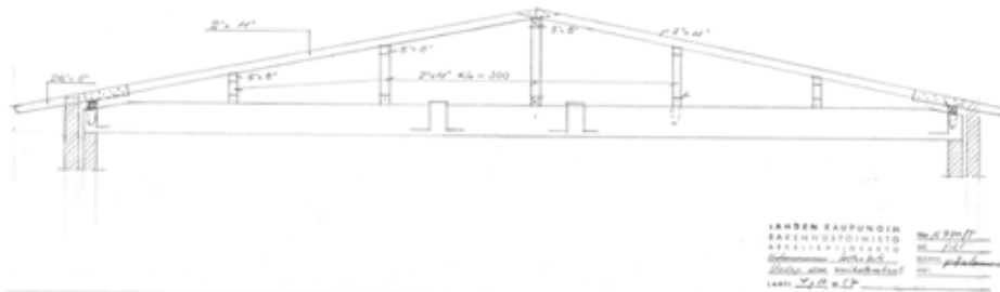
Kuva 60. Laajennuksen vesikattorakenteet. Piirustus on päivätty 4.10.1957. Kuva-lähde: Lahden Tilakeskus.
