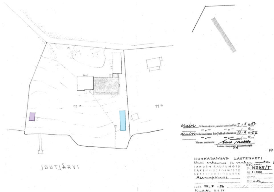
Kuva 49: Asemapiirros vuodelta 1957. Saunarakennus (korostettu violetilla) sijoittuu tontin länsirajalle rannan tuntumaan ja vaja (korostettu sinisellä) vastaavasti tontin itäpuolelle lähelle rantaa. Asemapiirustuksen, ilmakuviin ja vuodelta 1979 olevan valokuvan perusteella vajan kokoa on pienennetty vuoden 1957 jälkeen.
