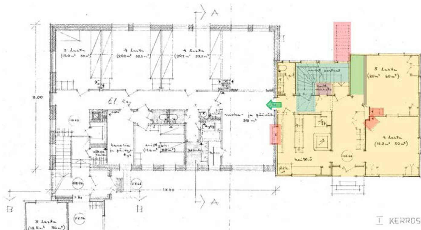
Kuva 123: Päärakennuksen ensimmäinen kerros (korostettu keltaisella) on kokenut useampia tilamuutoksia: Portaiden (sinisellä) suunta on muutettu, isommasta lastenhuoneesta on lohkaistu kylpyhuone (vihreällä) ja huoneen oviaukko on siirretty samaan linjaan toisen lastenhuoneen seinälinjan kanssa (harmaa viiva). Rakennuksen itäseinään on puhkaistu kulkuyhteys (vihreä nuoli) laajennusosaan. Lastenhuoneista on purettu tulisijat (punaisella). Samoin takapihan portaat ja uloskäynti sekä keittiön uloskäynti (punaisella) on poistettu käytöstä laajennusosan rakentamisen myötä. Keittiövarasto (violetilla) on muutettu wc-tilaksi. Kuva: Lahden Tilakeskus.
