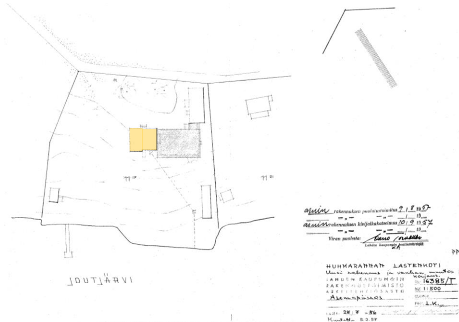
Kuva 31: Asemapiirros vuodelta 1957. Lastenkodin päärakennus (korostettu keltaisella) sijaitsee tontin keskellä, vuonna 1958 valmistunut lisäosa sen oikealla puolella ja vanhempi 1920-luvun taitteesta oleva sivuosa pohjoisempana kohtisuoraan Huhmarannankatua kohden. Rannan tuntumassa tontin länsilaidalla sijaitsee vanha saunarakennus ja itälaidalla varastorakennus. Alkuperäinen avokuisti huvilarakennuksen itäpäässä (merkitty katkoviivalla) joutui väistymään lisärakennuksen tieltä, samoin tapahihan portaat purettiin tai oli jo purettu asemapiirroksen laatimisen aikaan. Lähde: Lahden Tilakeskus.
