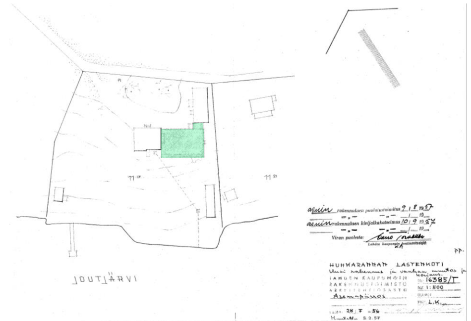
Kuva 37: Asemapiirros vuodelta 1957. Massaltaan muita rakennuksia suurempi lisäosa (korostettu vihreällä) on rakennettu kiinni kahteen tontin alkuperäiseen rakennukseen siten, että ne yhdessä muodostavat L-kirjaimen muotoisen kokonaisuuden. Kolmen rakennuksen muodostama massa erottaa myös tontin etu- ja takapihat selkeämmin toisistaan verrattuna aiempaan tilanteeseen, jossa tontilla olivat vain alkuperäiset Huhmarannan huvilan aikaiset puurakennukset. Lähde: Lahden Tilakeskus.
