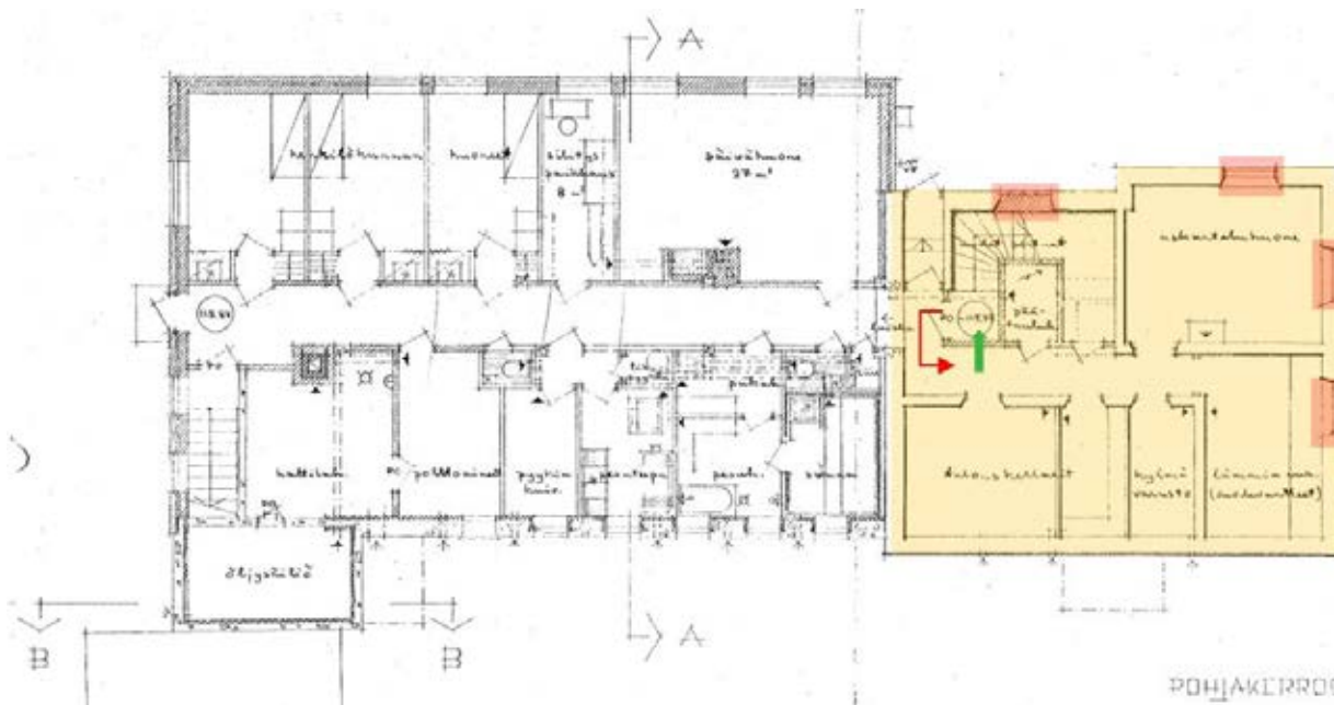
Kuva 119: Ote vuoden 1957 pohjapiirustuksesta. Päärakennuksen kellarikerros on korostettu keltaisella. Umpeen muurattut ikkunat on osoitettu punaisella ja portaikon oven vanha paikka punaisella ja uusi sijainti vihreällä nuolella. Lähde: Lahden Tilakeskus.
