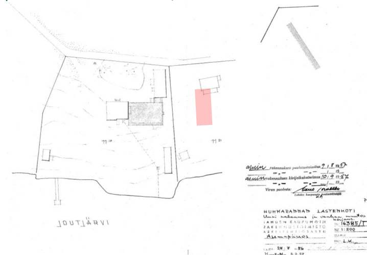
Kuva 35: Asemapiirros vuodelta 1957. Vanha 1920-luvun taitteesta oleva asuinrakennus (korostettu punaisella) sijaitsee tontin pohjoisosassa lähes kohtisuoraan Huhmarannankatua. Asemapiirroksessa rakennuksen kaksi sisäänkäyntiä on osoitettu, mutta pienempi niistä poistuvana/poistettuna rakenteena. Lähde: Lahden Tilakeskus.
