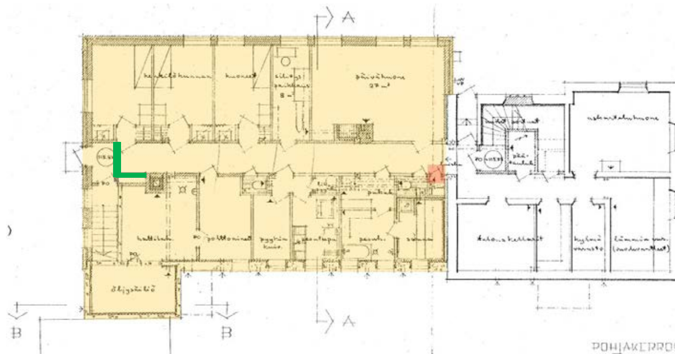
Kuva 151: Laajennusosan kellarikerros (korostettu keltaisella) on säilynyt tilajaan osalta pitkälti alkuperäisen mukaisena. Portaikko on palo-osastoitu uudelle seinäpätkällä ja metallipalo-ovella. Myös itäpäädyn käytävän seinälinja on suoristettu (vihreällä korostetut osat). Siivouskomeron ovea (punaisella) ei enää ole. Kuva: Lahden Tilakeskus.
