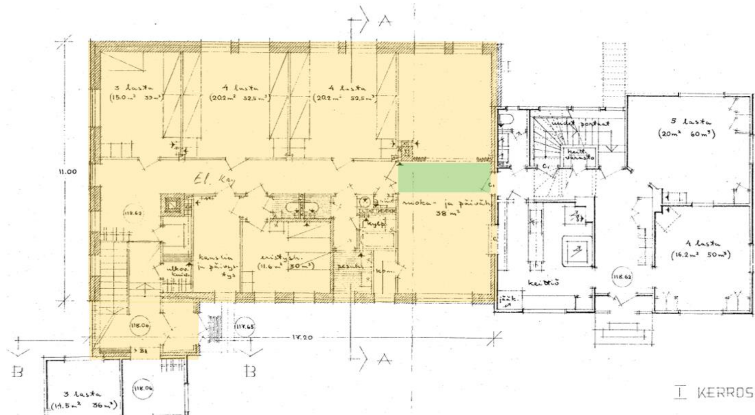
Kuva 163: Laajennusosan ensimmäinen kerros (korostettu keltaisella) on säilynyt tilajaon osalta alkuperäisen pohjapiirroksen mukaisena. Huomiota herättävin muutos on päivähuoneen katon alaslasku kookkaan ilmanvaihtokanavan kohdalla (merkitty vihreällä). Kuva: Lahden Tilakeskus.
