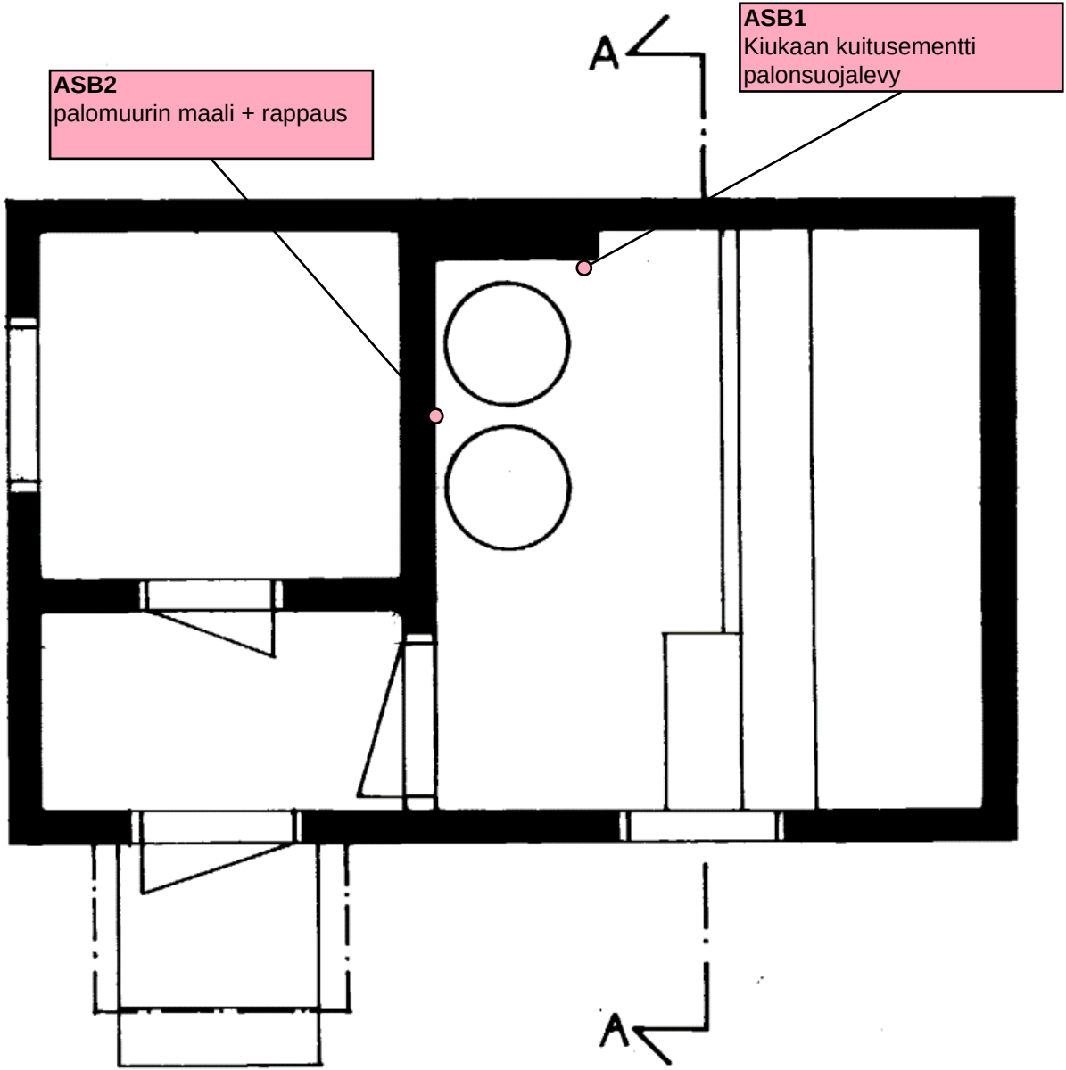
POHJA 1:50
