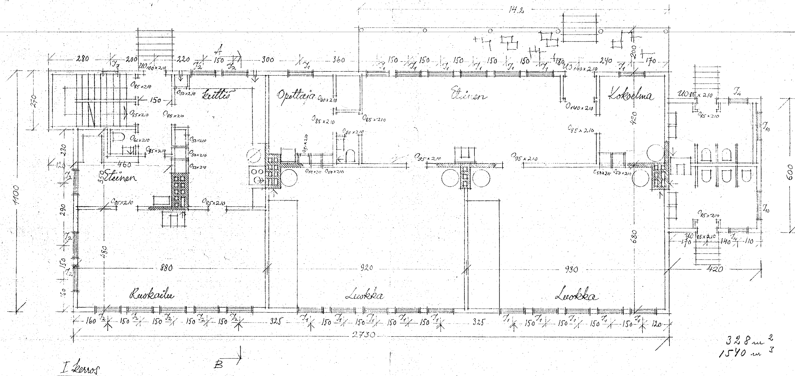
Kuva 9: Pohjapiirustus, 1.krs 1947. 1:100 (kuvaa rajattu).
