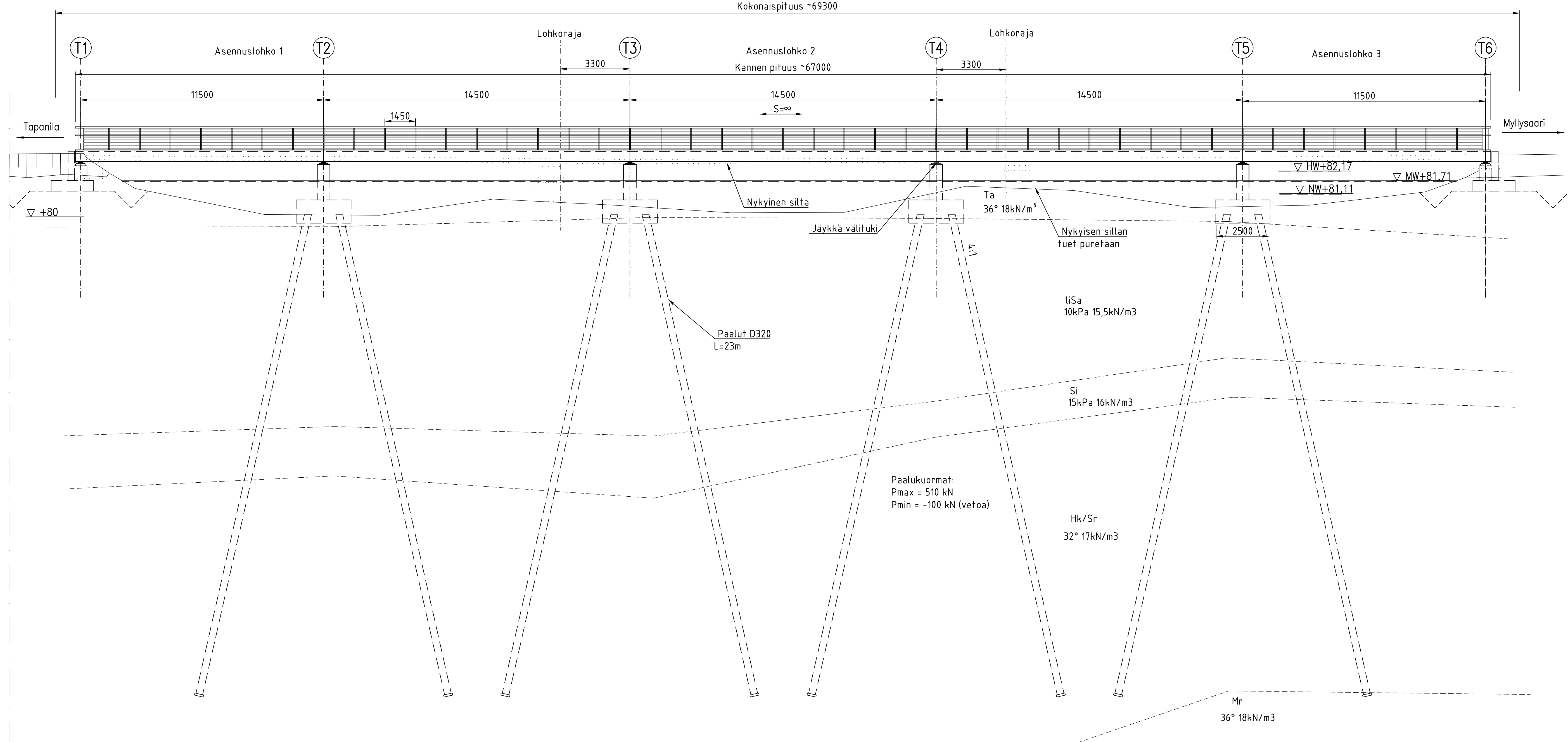
A-A 1:100
