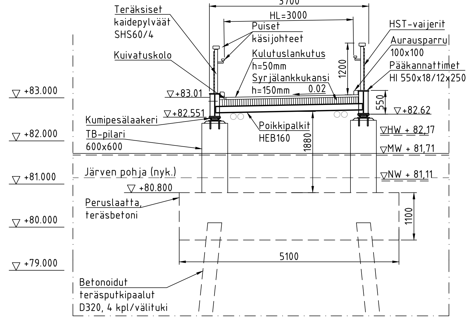
B-B 1:50
