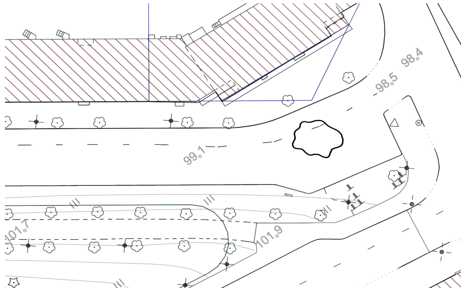
VIISKULMAN AUKIO TYYPIPOIKKILEIKKAUS A-A 1:100
