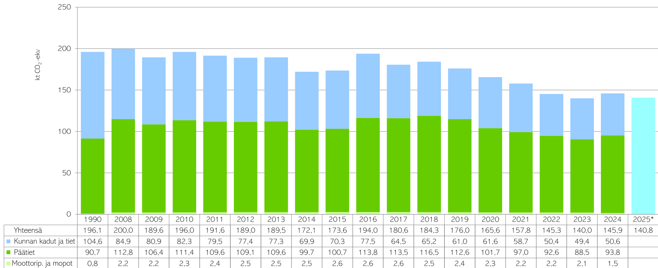
Kuva 7. Tieliikenteen päästöt Lahdessa vuonna 1990 ja vuosina 2008–2025. Vuoden 2025 tieto on ennakkotieto. (CO2-raportti, 2026)
