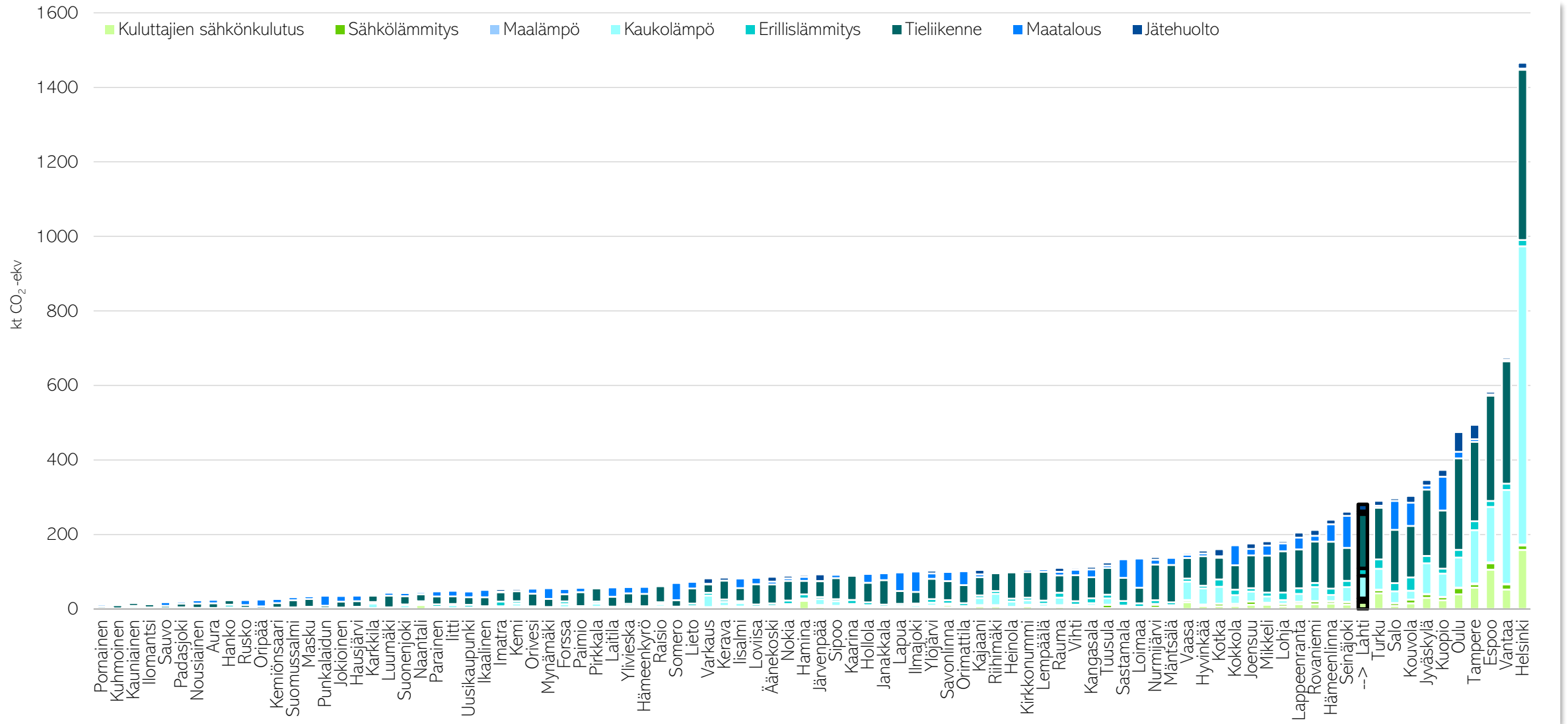
Kuva 19. Kokonaispäästöt (kt CO 2 -ekv) kaikissa CO 2 -raportin kunnissa vuonna 2024 ilman teollisuutta ja muita liikennemuotoja. (CO 2 -raportti, 2026)
