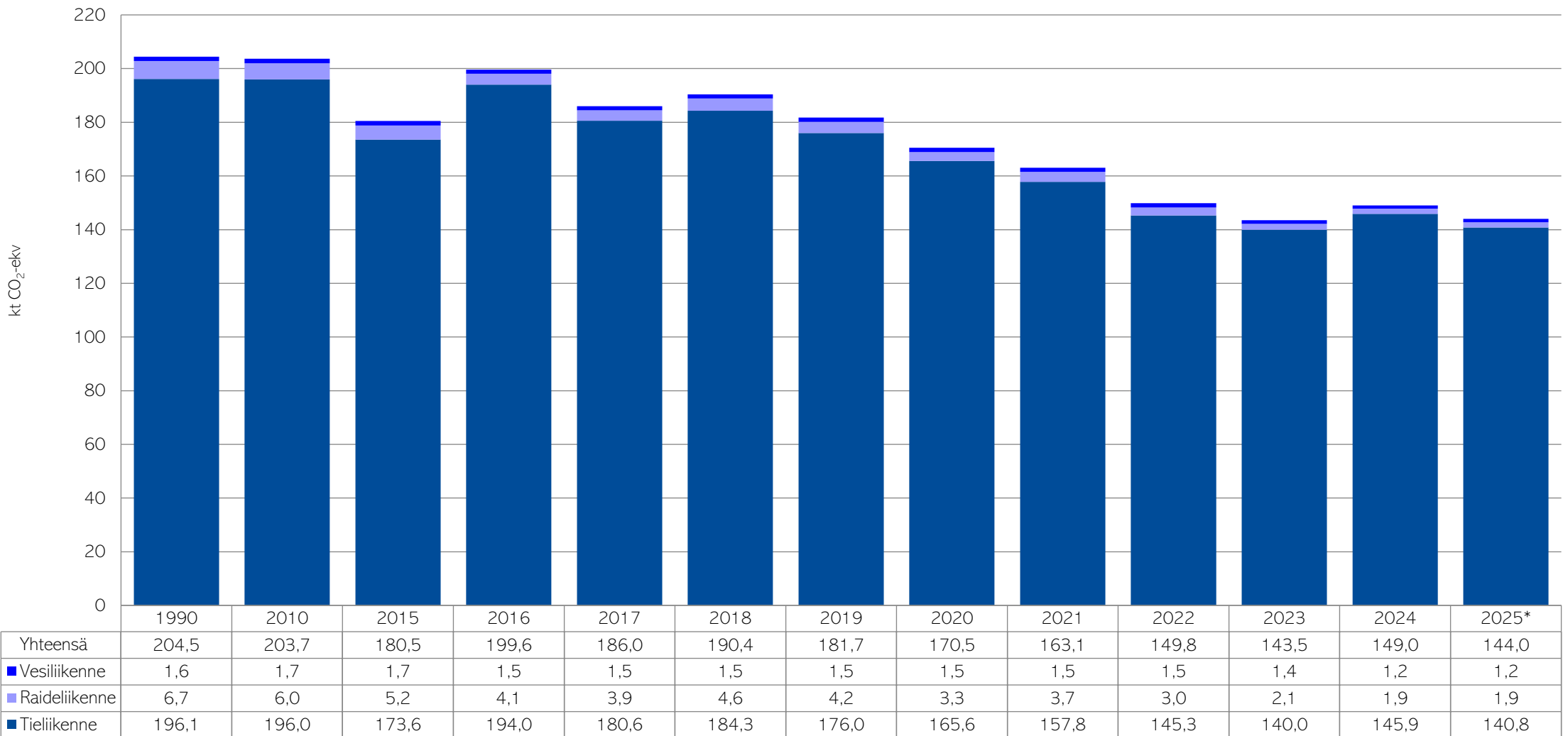
Kuva 8. Kaikkien liikennemuotojen päästöt yhteensä Lahdessa vuosina 1990, 2010 ja 2015–2025. Vuoden 2025 tiedot ovat ennakkotietoja. (CO 2 -raportti, 2026).
